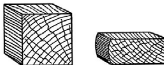
Рис. 3.4. Деревянный образец до и после сжатия поперек волокон
