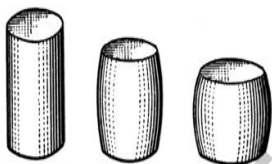
Рис. 3.1. Деформация стального образца при сжатии
