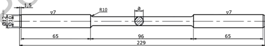
Рис. 4.5. Образец для испытания на усталость при чистом изгибе
