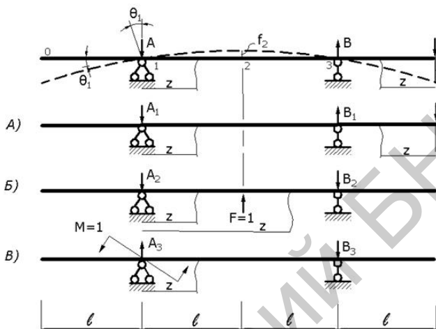
Рис. 7.1. Расчетная схема балки
