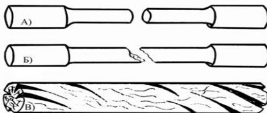
Рис. 5.1. Характер разрушения образцов при кручении: а – разрушение стального образца, вызванное сдвигом по поперечному сечению образца; б – разрушение чугунного образца от отрыва по винтовой поверхности с углом наклона 45^\circ к оси образца; в – разрушение деревянного образца, вызванное сдвигом в продольном осевом сечении
