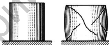
Рис. 3.2. Деформация чугунного образца при сжатии
