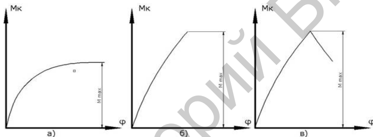
Рис. 5.2. Диаграмма кручения образцов: а – стального; б – чугунного; в – деревянного
