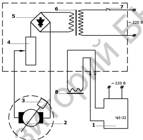
Рис. 8.1. Электрическая схема экспериментальной установки:
