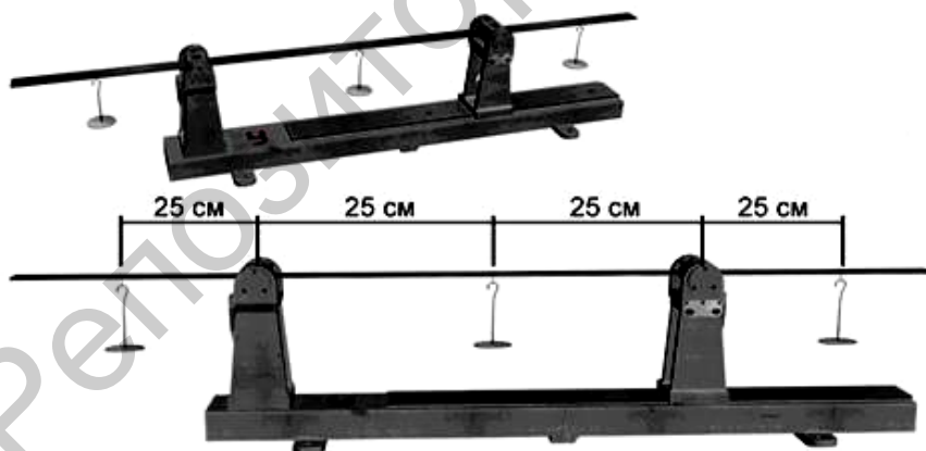
Рис. 7.2. Установка СМ-4А
